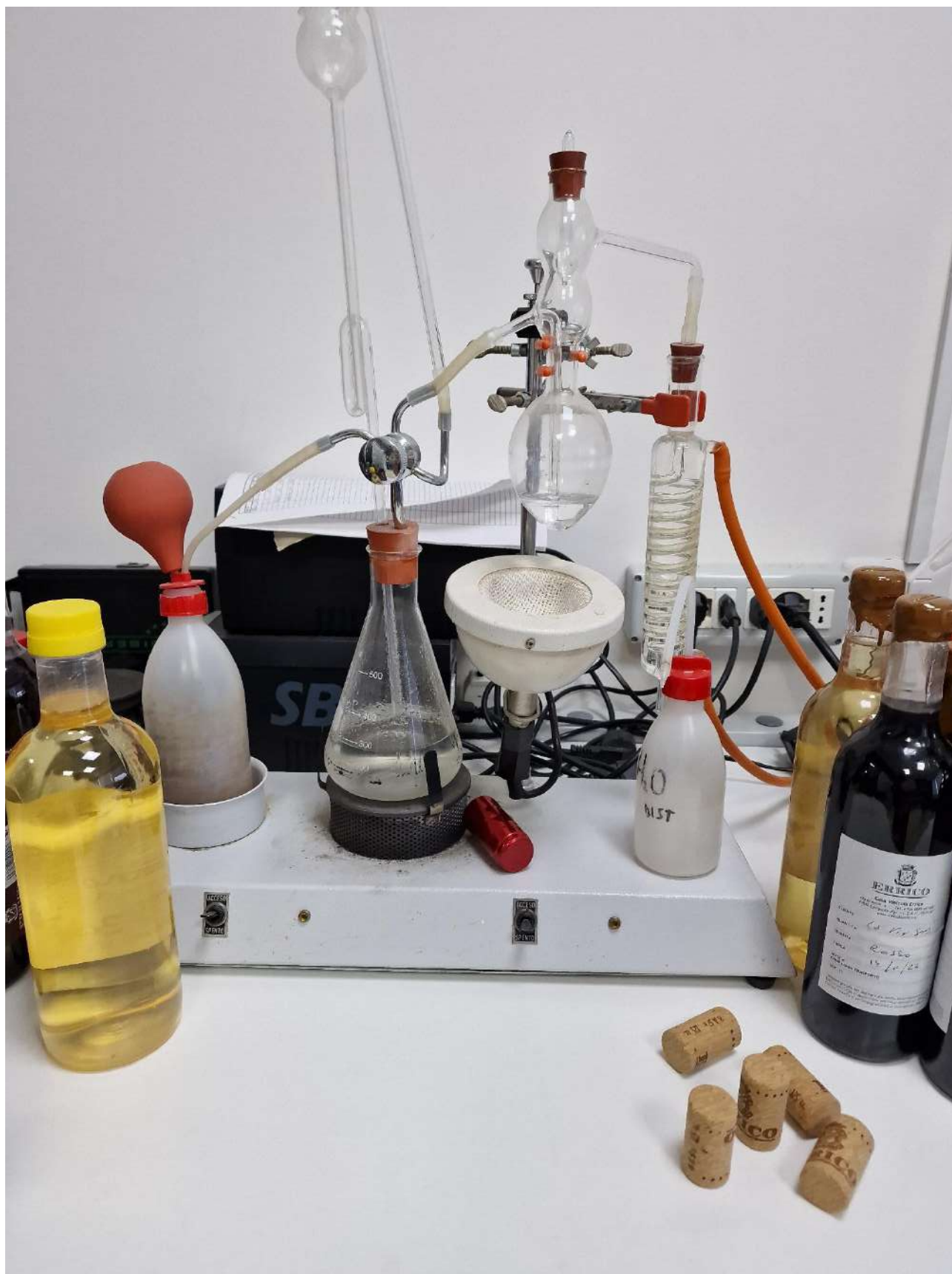
65- DISTILLATORE ENOMICO, ACIDIMETRO GIBERTINI
