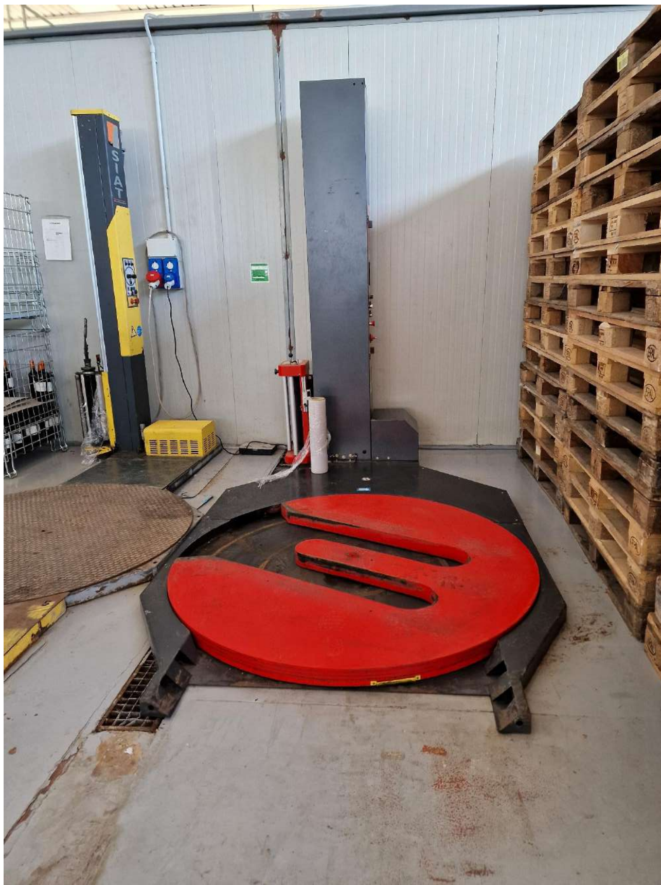
14-IMBALLATORE AUTOMATICO
